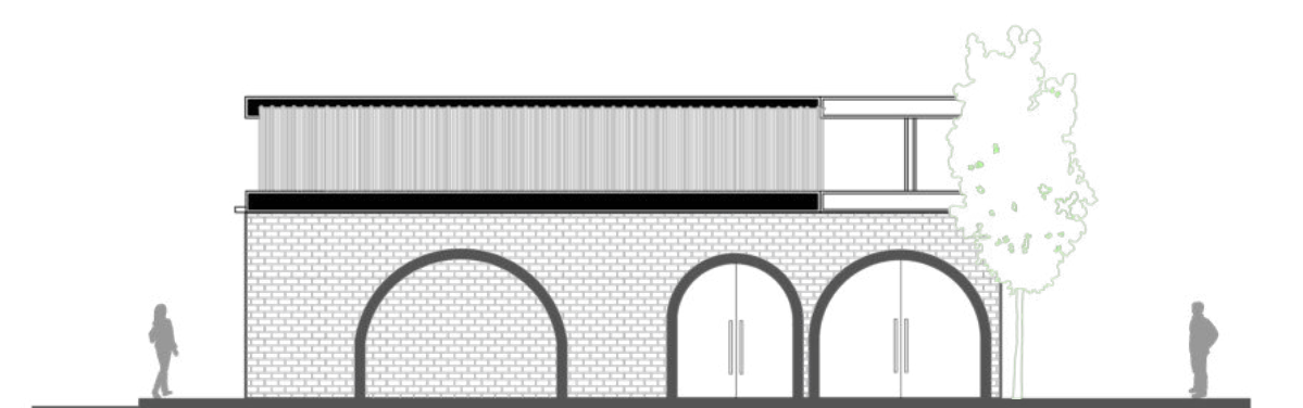
FACHADA SUR / MANZANA
