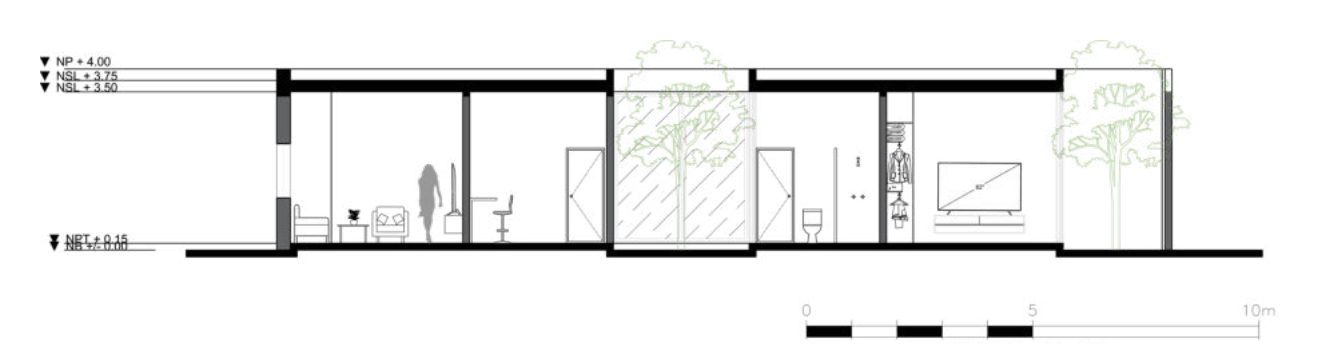
CORTE LONGITUDINAL / MANZANA
