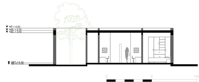
CORTE TRANSVERSAL / MANZANA
