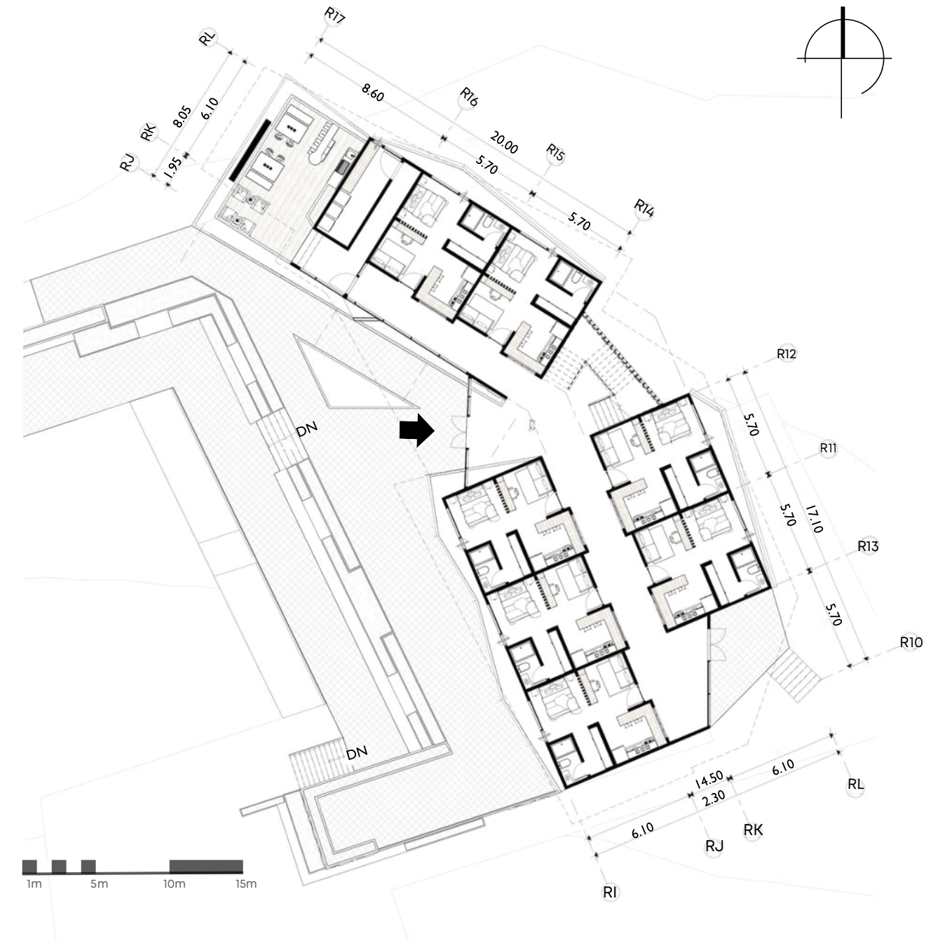
PLANTA TIPICA-ED. PROFESORES
