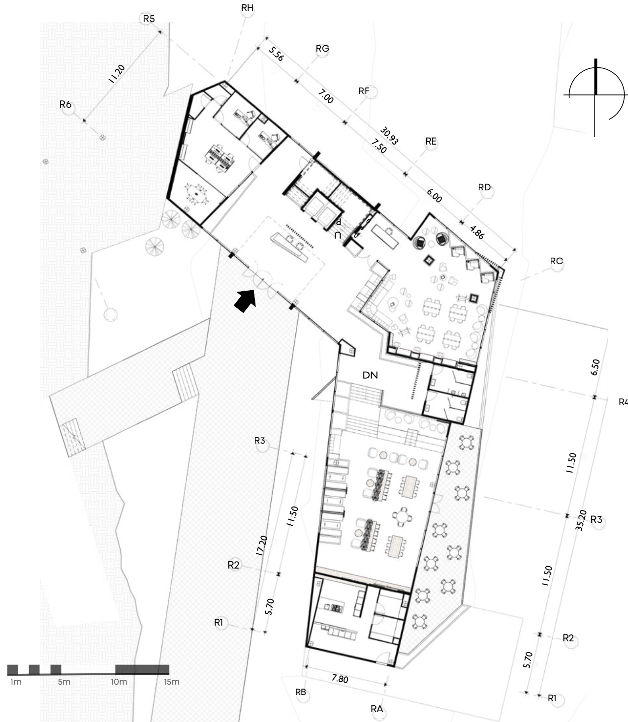
PLANTA NIV. 1-ED. ESTUDIANTES
