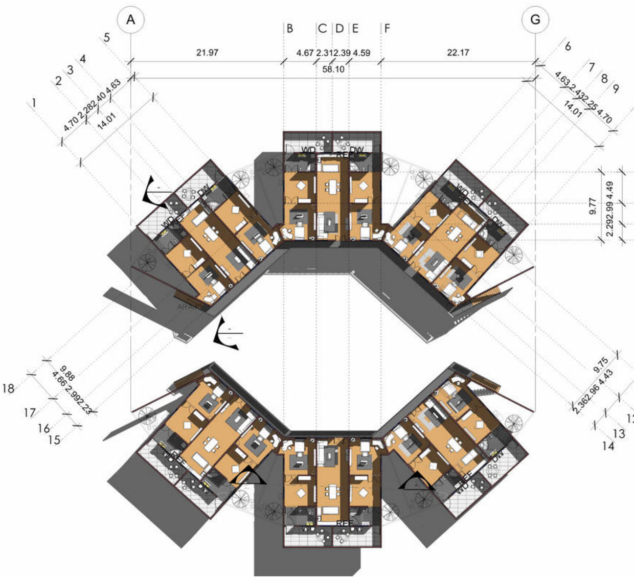
Planta alta Residenciales
