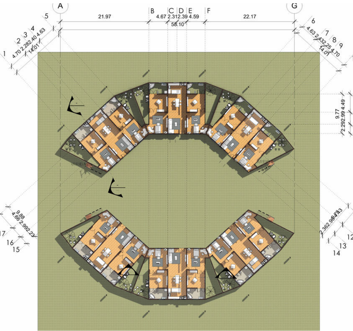
Planta baja Residenciales
